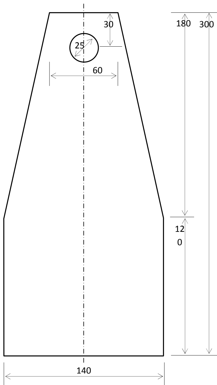
Obrázek č.3 - boční stěna (tl. 17 mm) - 2 kusy
